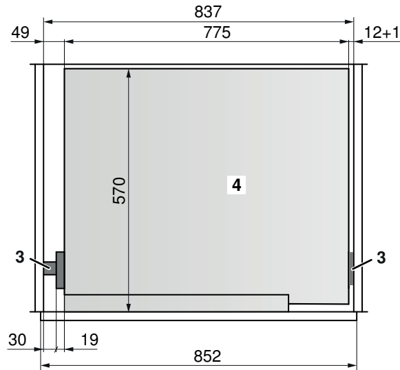
Plan au sol
